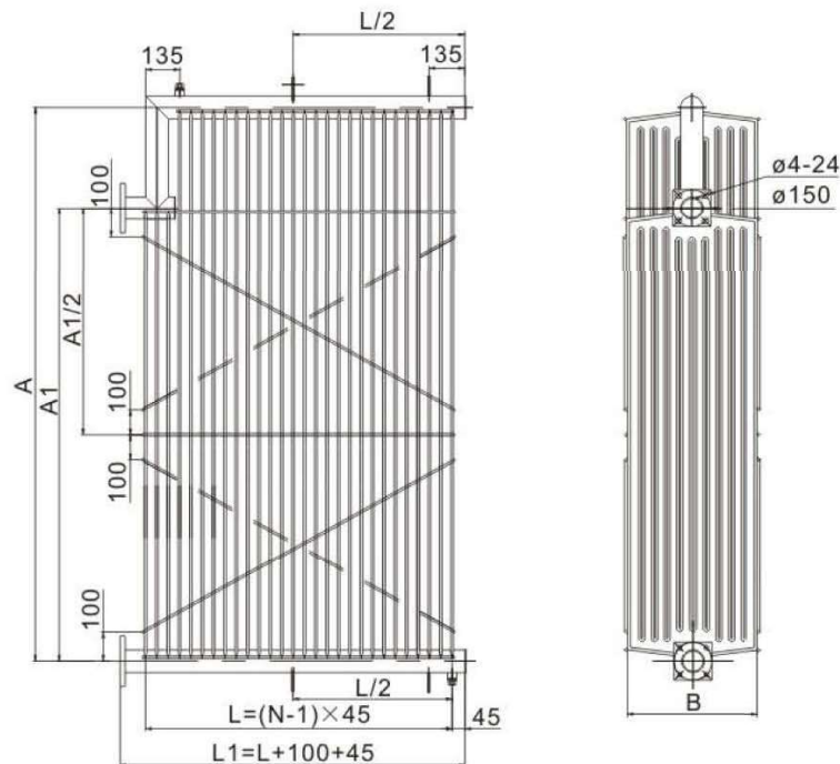
PCJ型片式散热器 (图2) PCJ type sheet radiator (Fig. 2)
